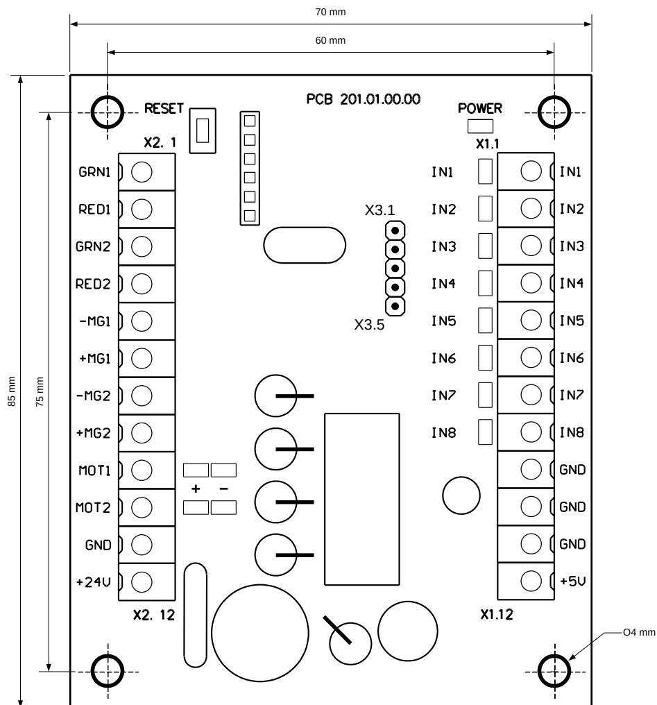
Рисунок 2 – Внешний вид контроллера моторизированного механизма РСВ.201.01.00.00
