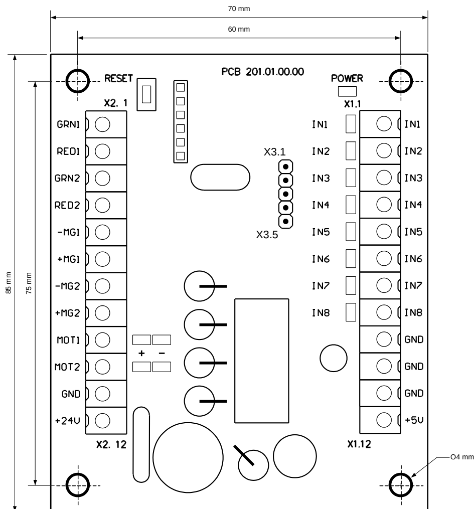
Рисунок 2 – Внешний вид контроллера РСВ.201.01.00.00
