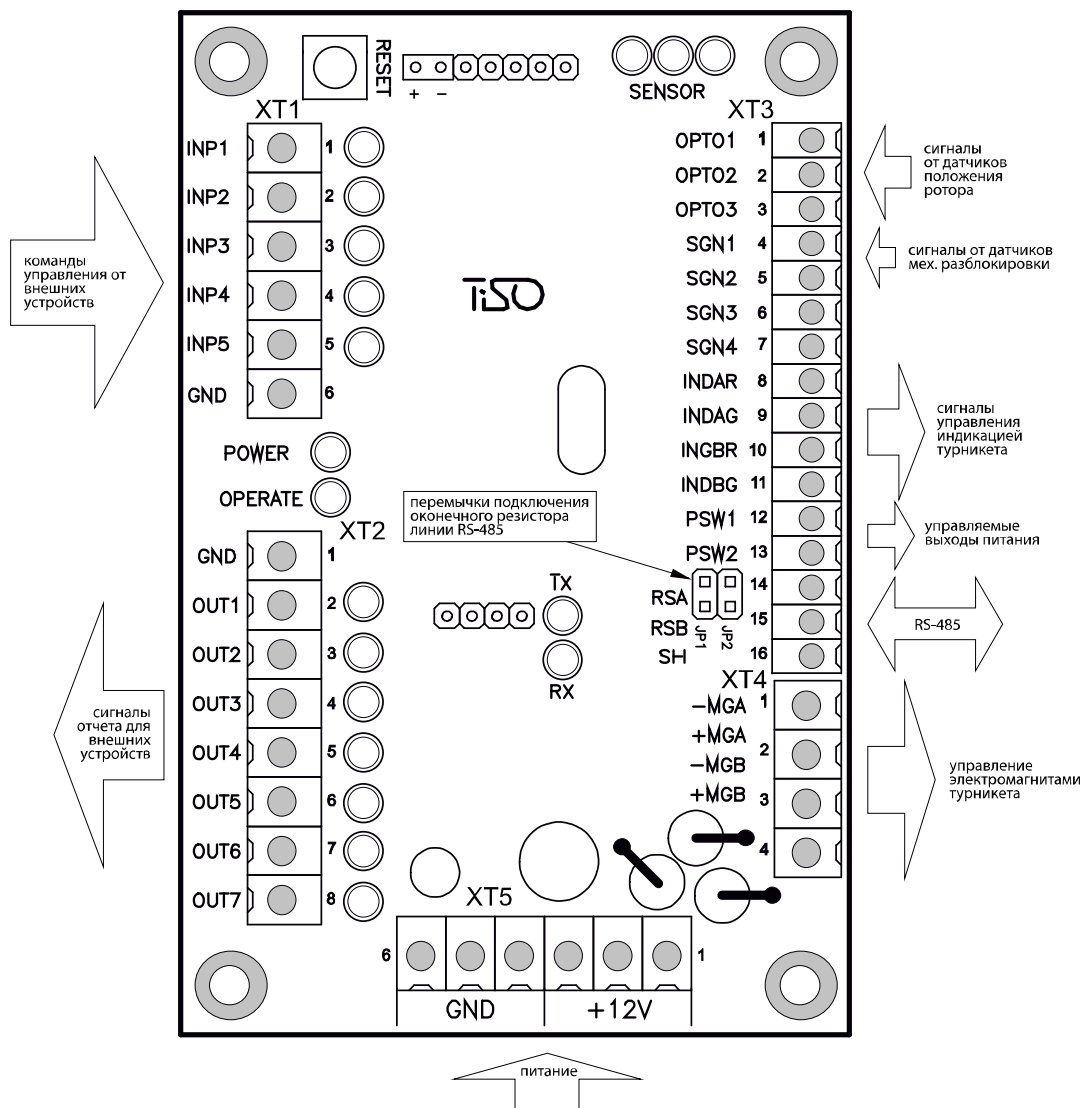
Рисунок 3 – Внешний вид контроллера РСВ.112.21.20.00
